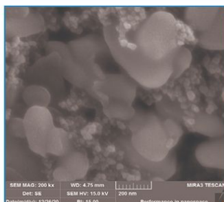
شکل ۱۰- رنگ فوق آب‌گریز ژیکالر با بزرگنمایی ۲۰۰ هزار
